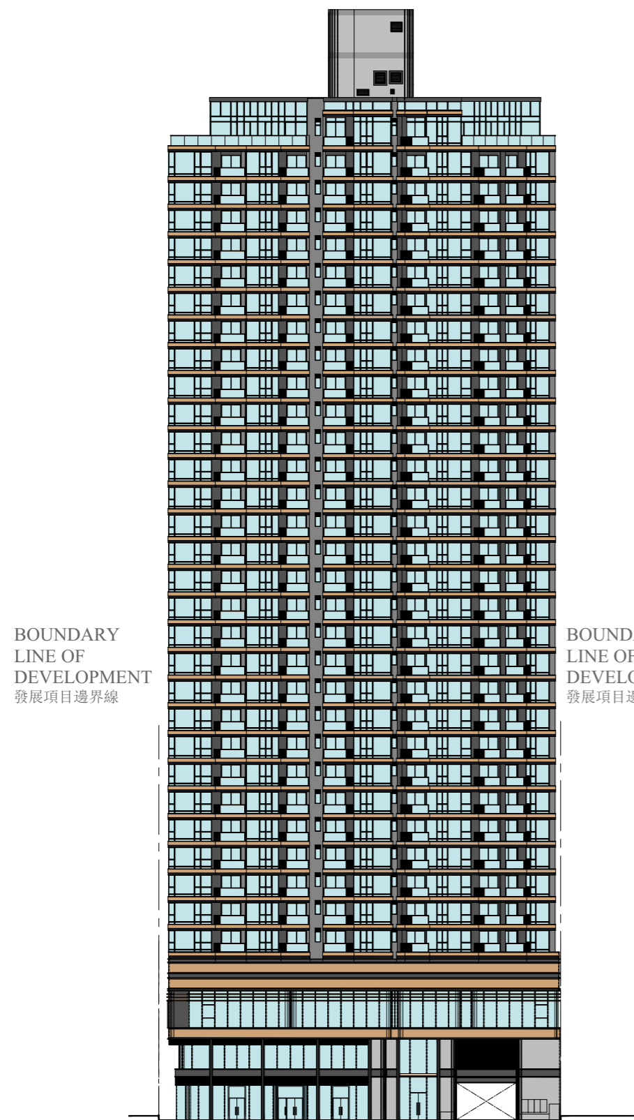
ELEVATION A 立面圖 A
